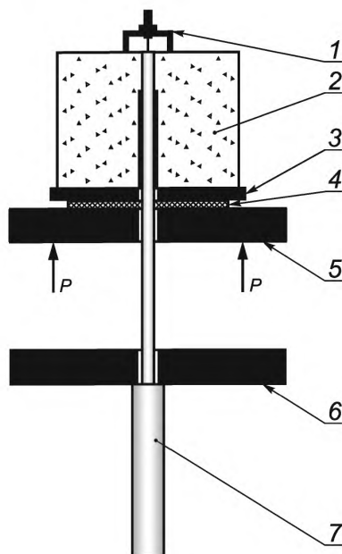
Рисунок 9.3 — Схема испытания образца при осевом выдерживании из бетонного куба
