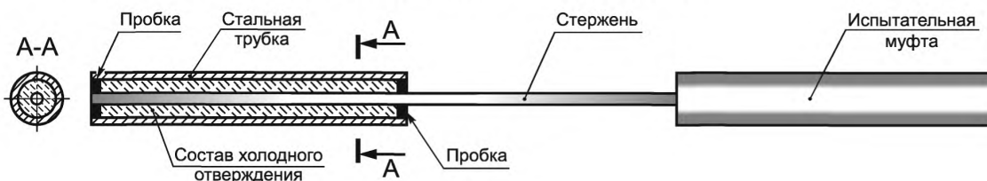
Рисунок 6.1 — Вид типового опытного образца
