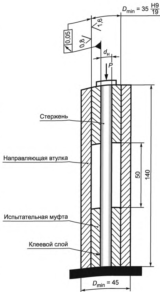
Рисунок 7.2 — Приспособление для испытания образцов на сжатие
